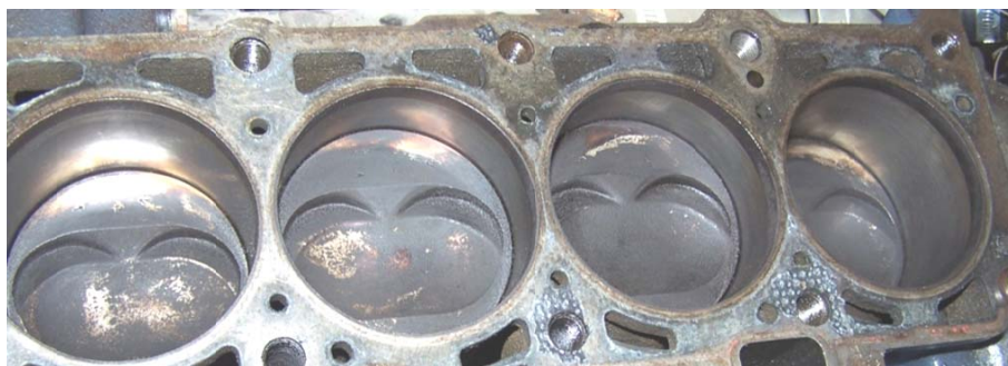
Рисунок 7 Внешний вид камеры сгорания со стороны блока цилиндров после работы двигателя на топливно-водной смеси
